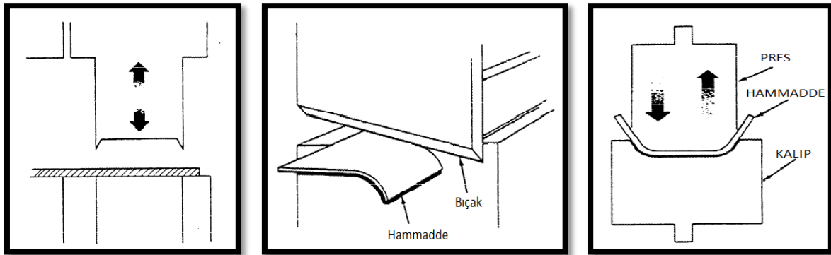
Şekil 11. Kopma ve ezilme tehlikelerinin bulunduğu hareketler [8]
