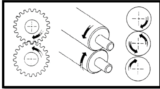
Şekil 6. Döner parçalar için sıkıştırma noktalarına örnekler [8]
