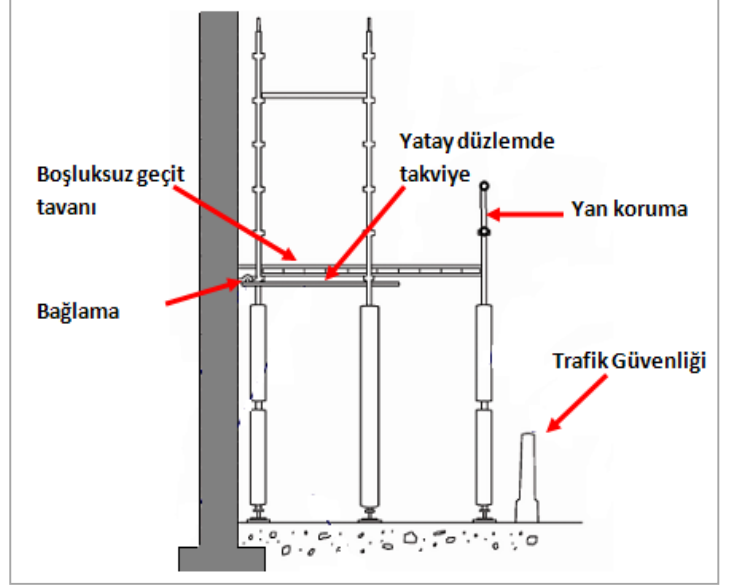
Şekil 36: Yaya geçidi
