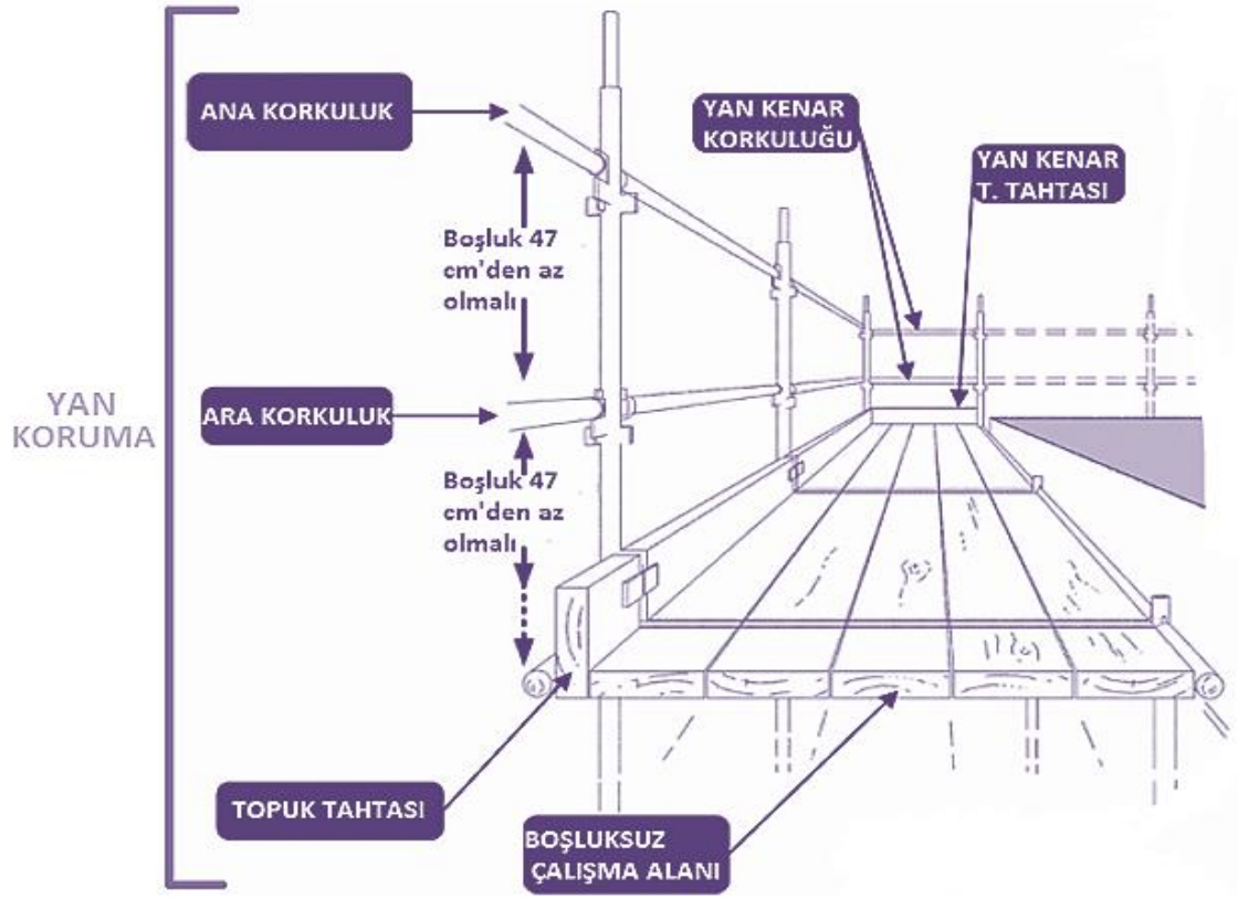
Şekil 7: Yan koruma
